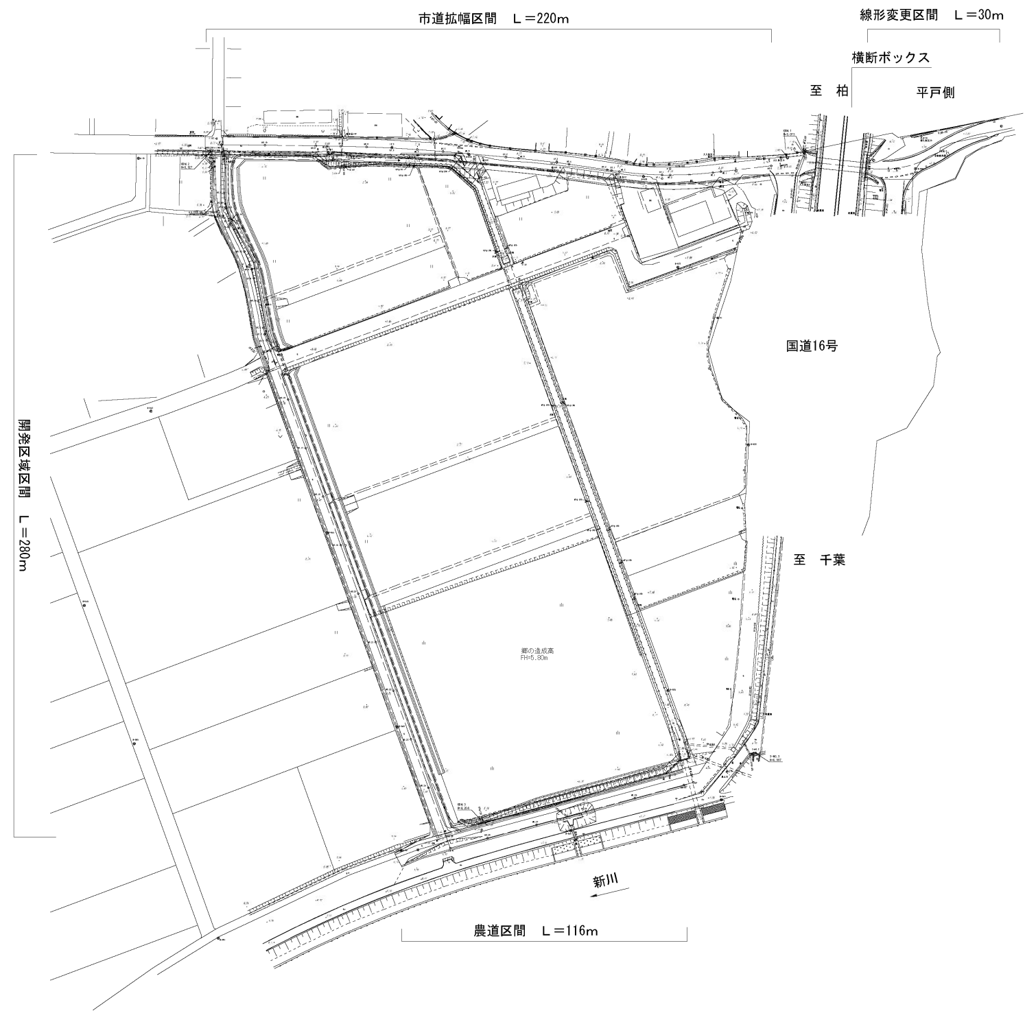
平面図
