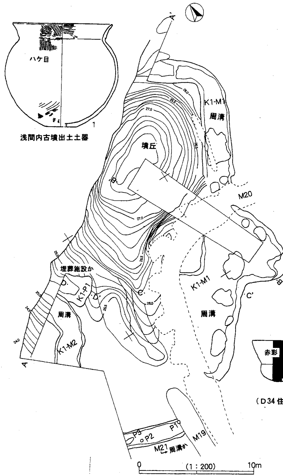
K1古墳(浅間内古墳)実測図
