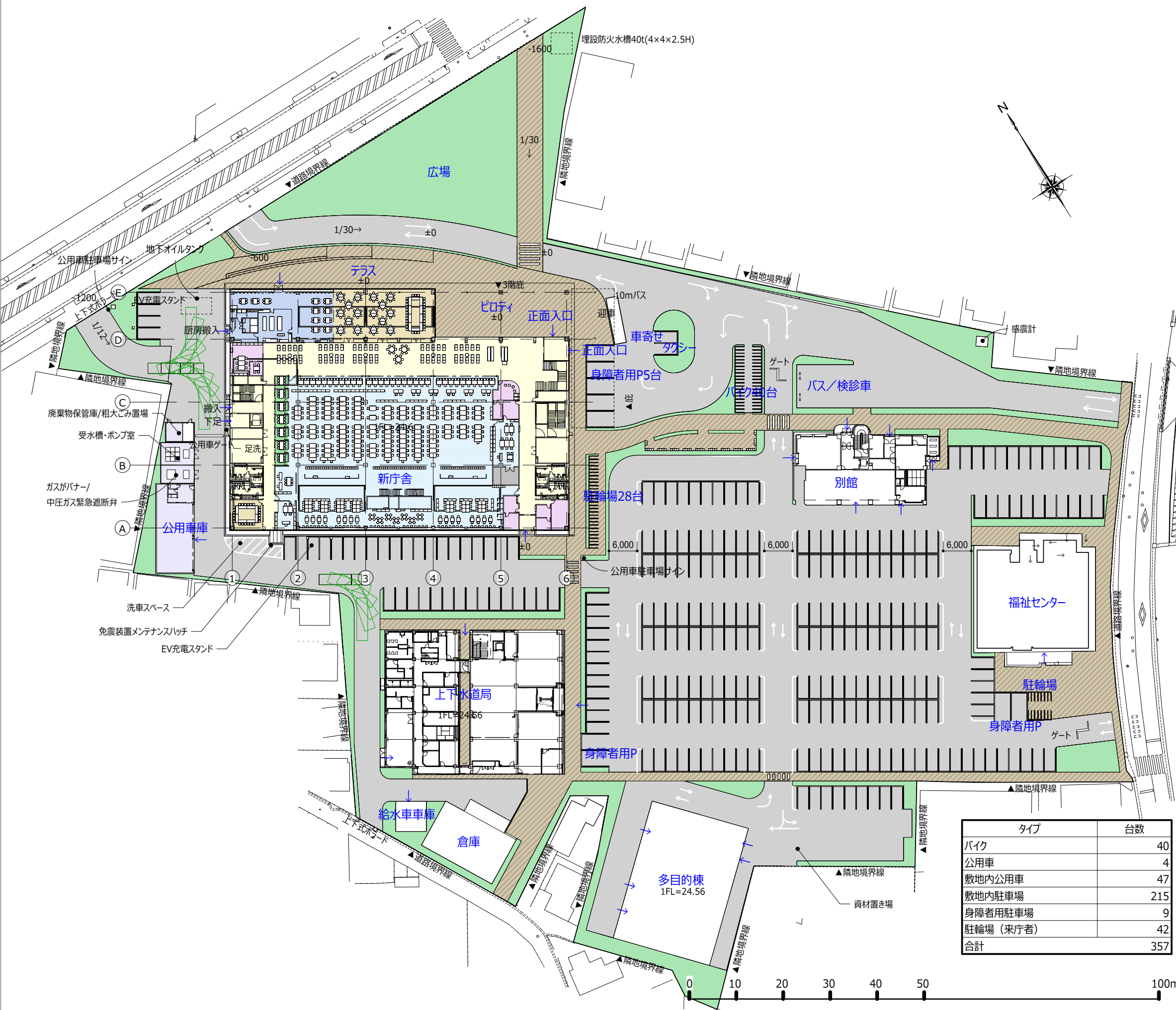
配置図
