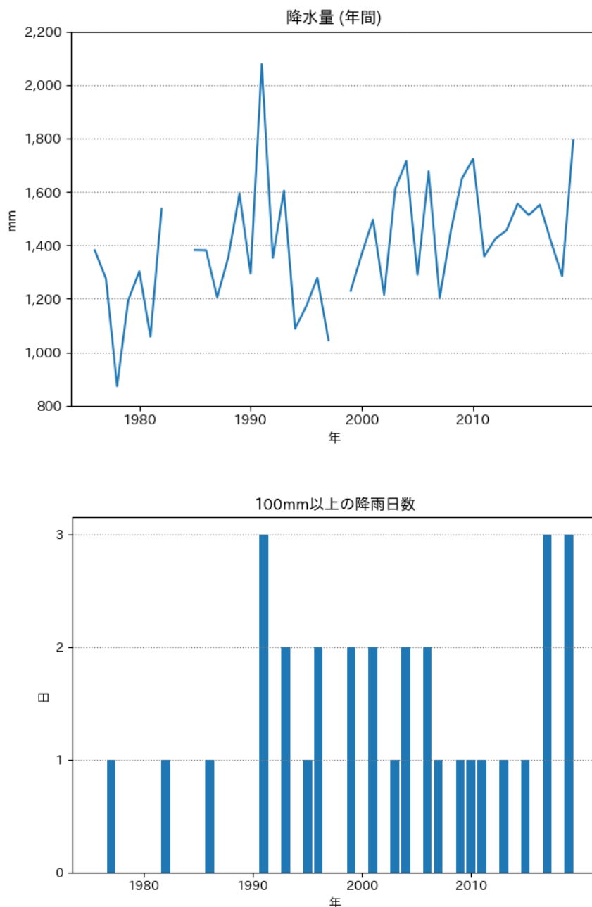
年間降水量・100 mm以上の降雨日数の推移(佐倉観測所)
