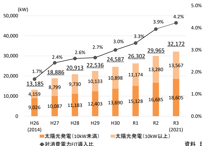
図 市域の再生可能エネルギーの導入容量累積の経年変化
