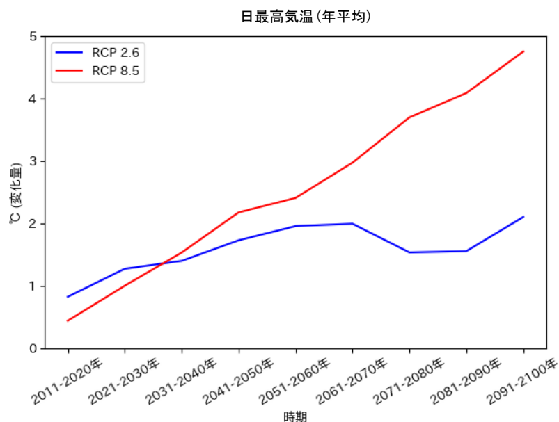
年平均気温・日最高気温(年平均)の推移予測(八千代市)
