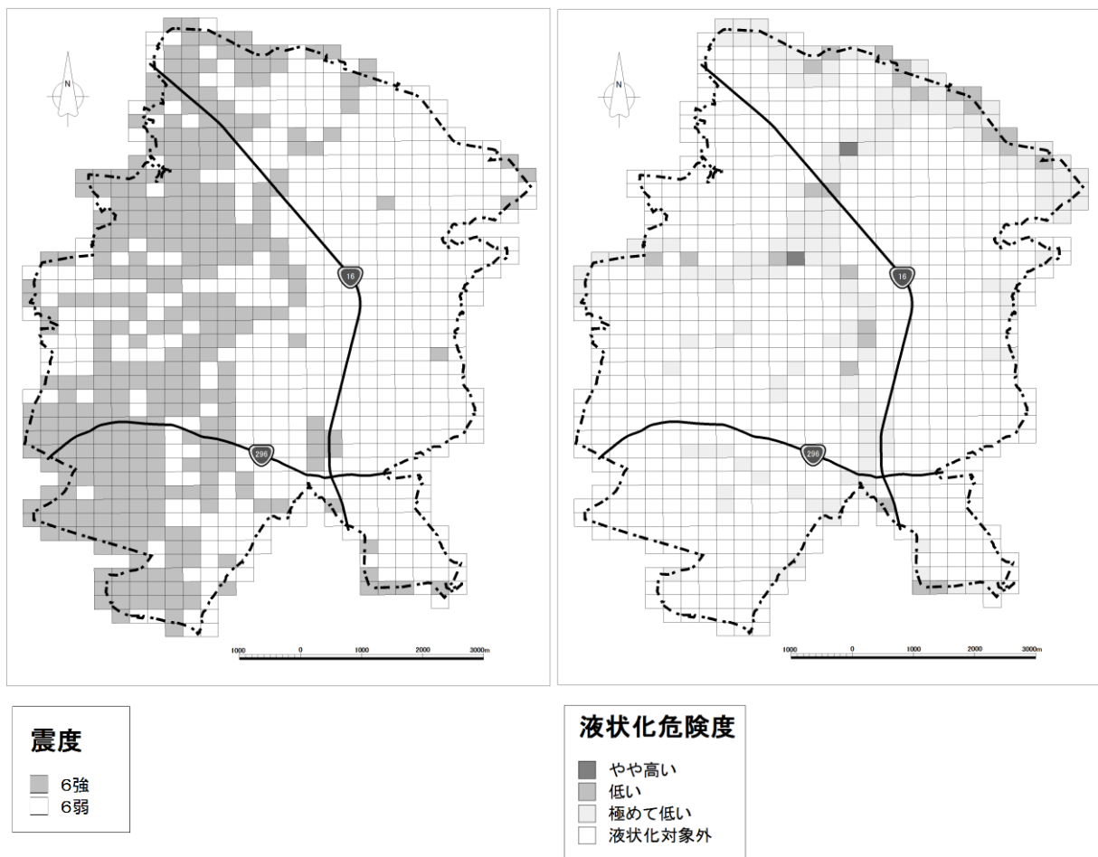
千葉県北西部直下地震の予測
