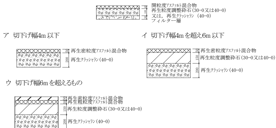
図3-5 歩道の設計例
