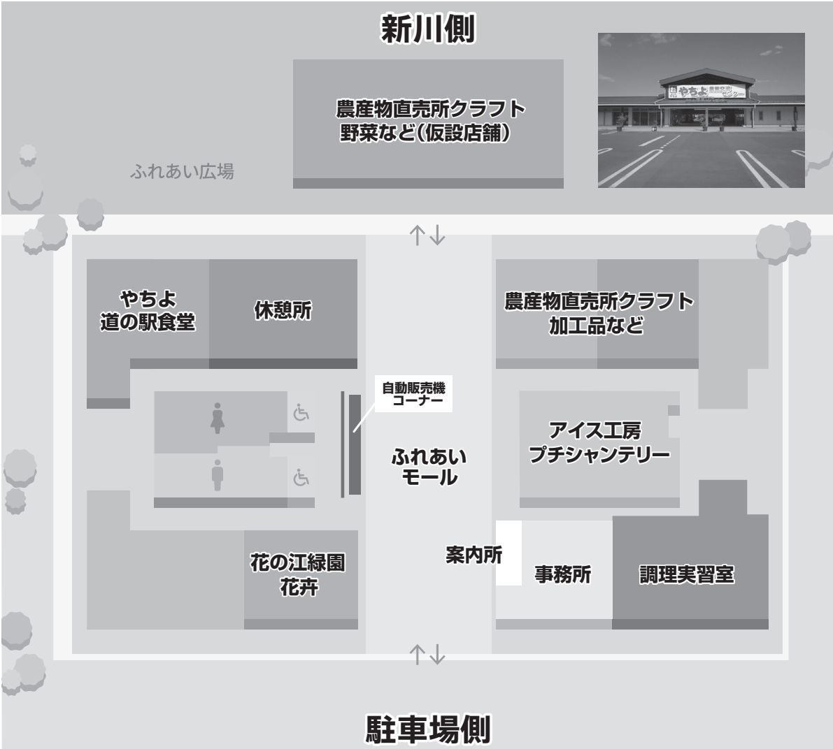
■やちよ農業交流センター機能移転後の施設レイアウト
