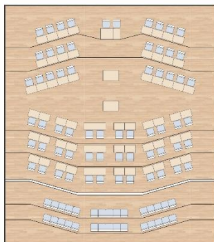
図 12 議場イメージ(左:レイアウトイメージ 右:断面イメージ)
