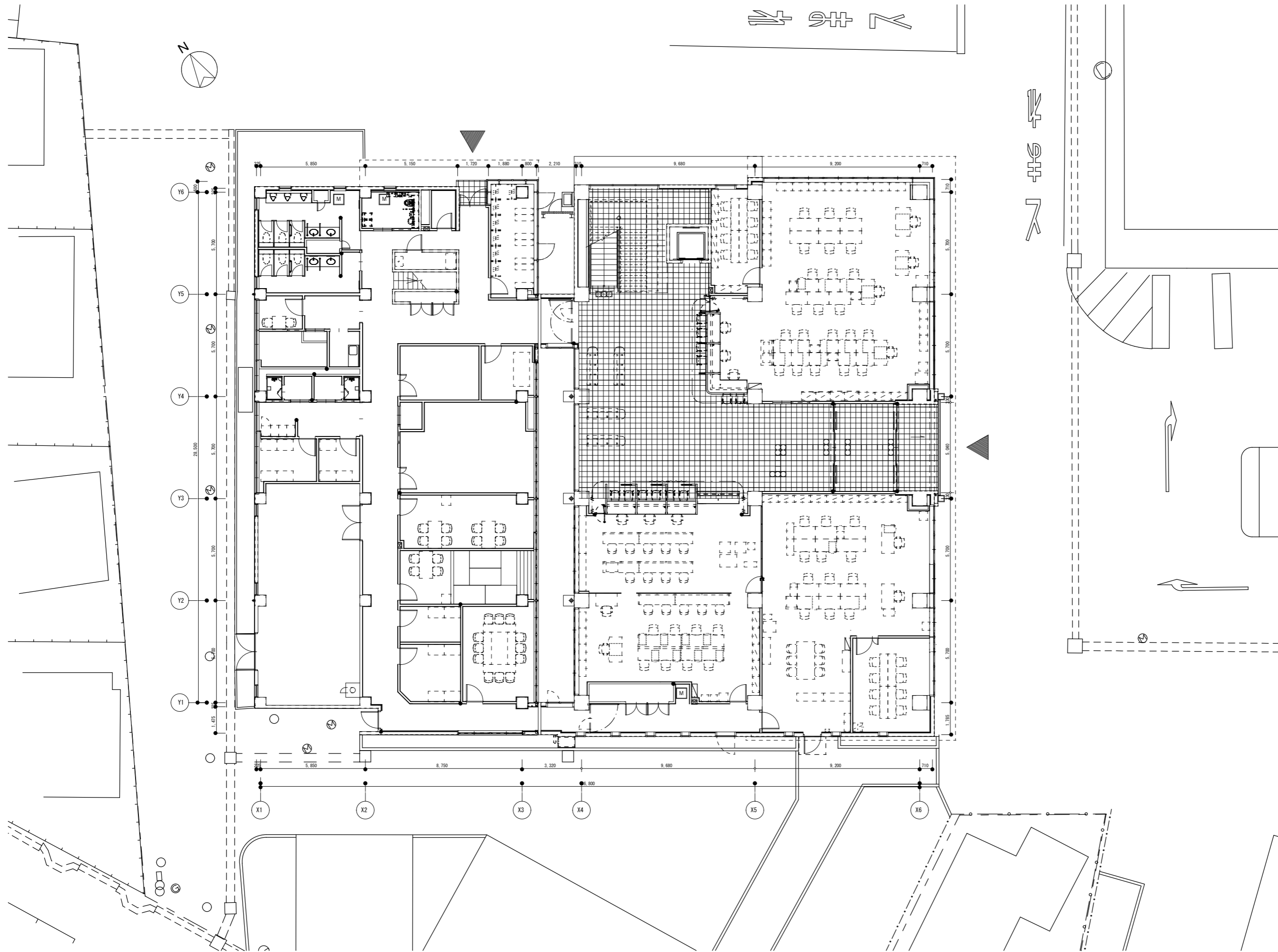
上下水道局庁舎 1階平面図
