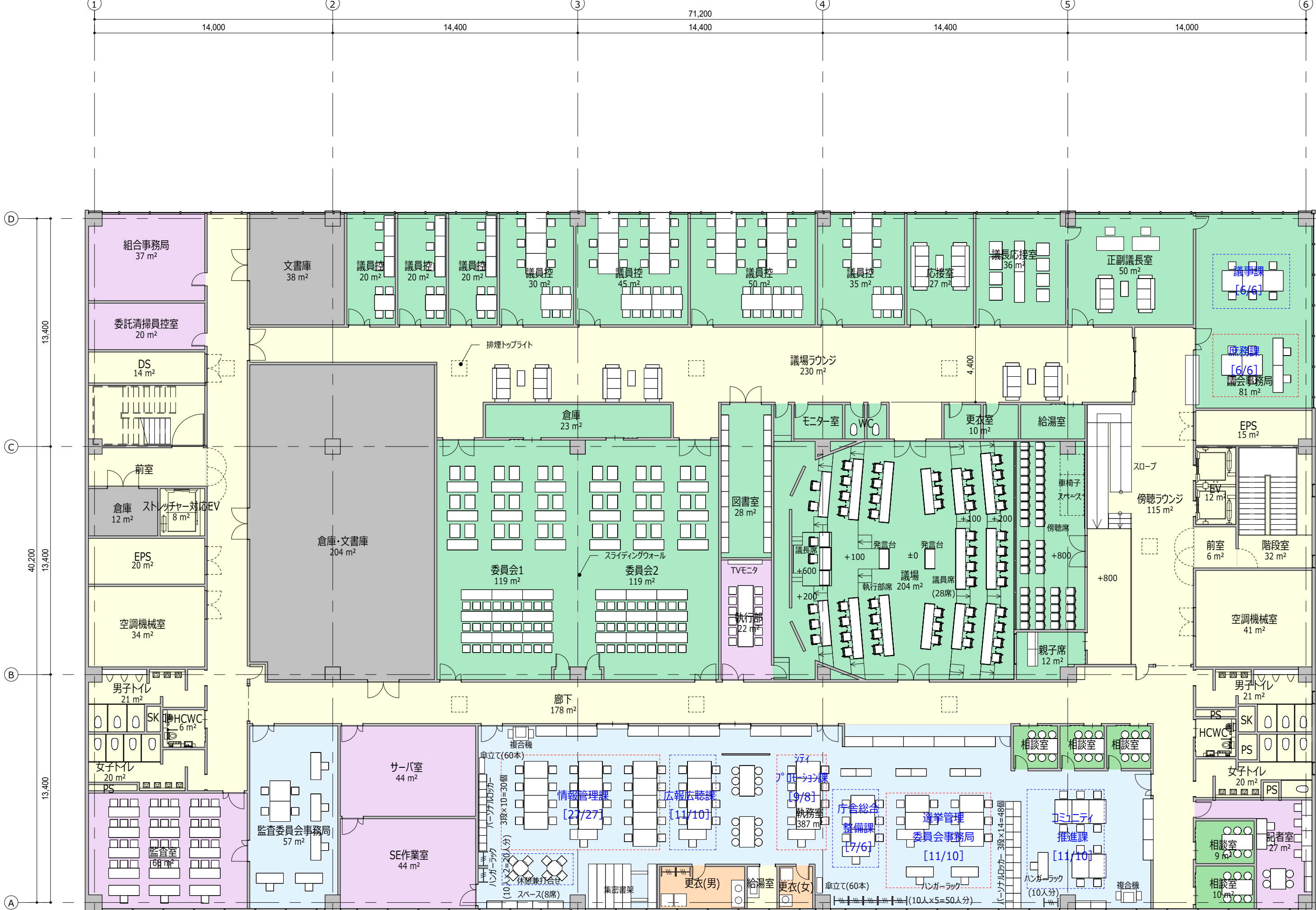
■ 4階平面図 2,950m 2 A3:1/200
