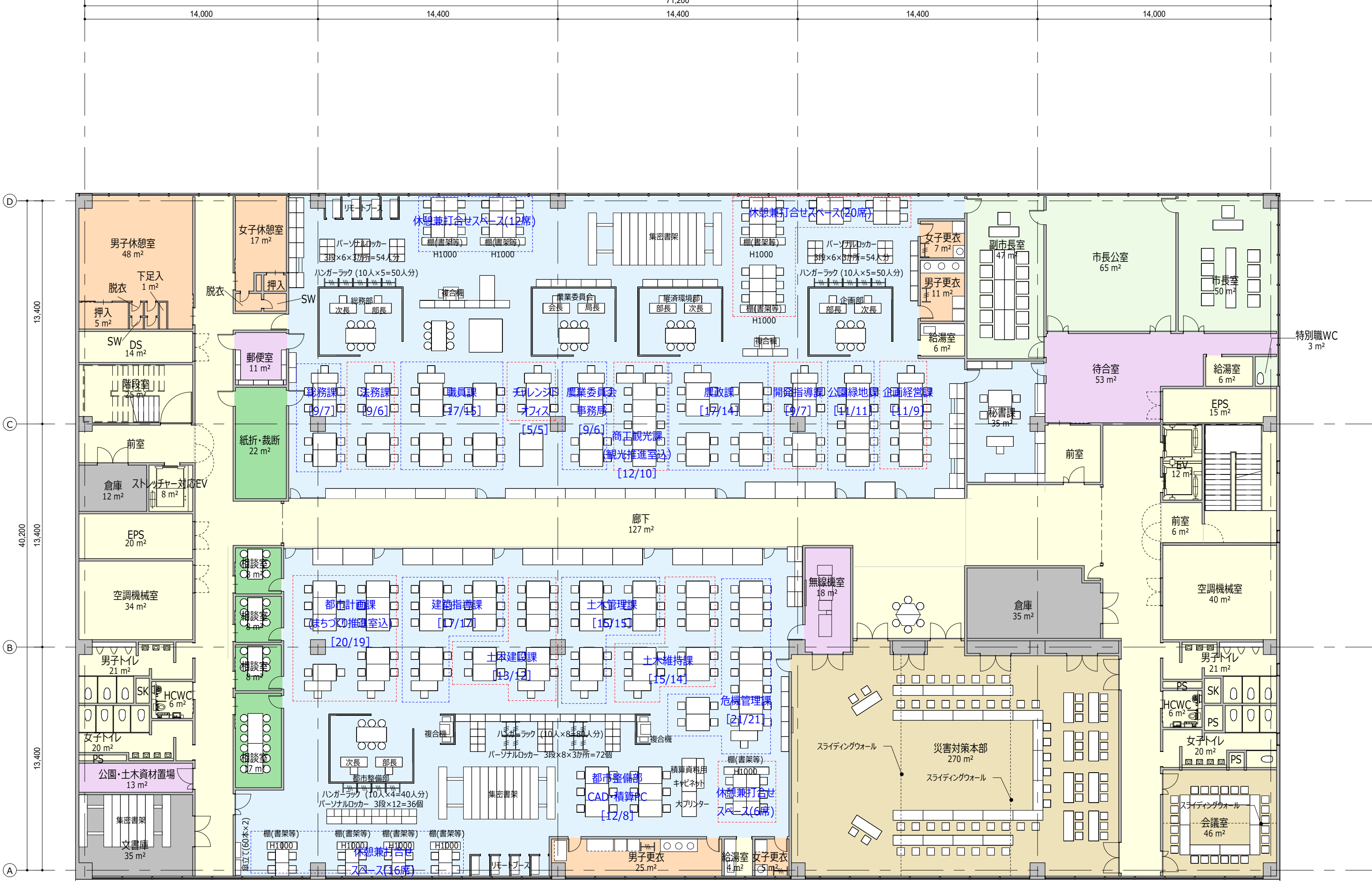
■ 3階平面図 2,950㎡ A3:1/200
