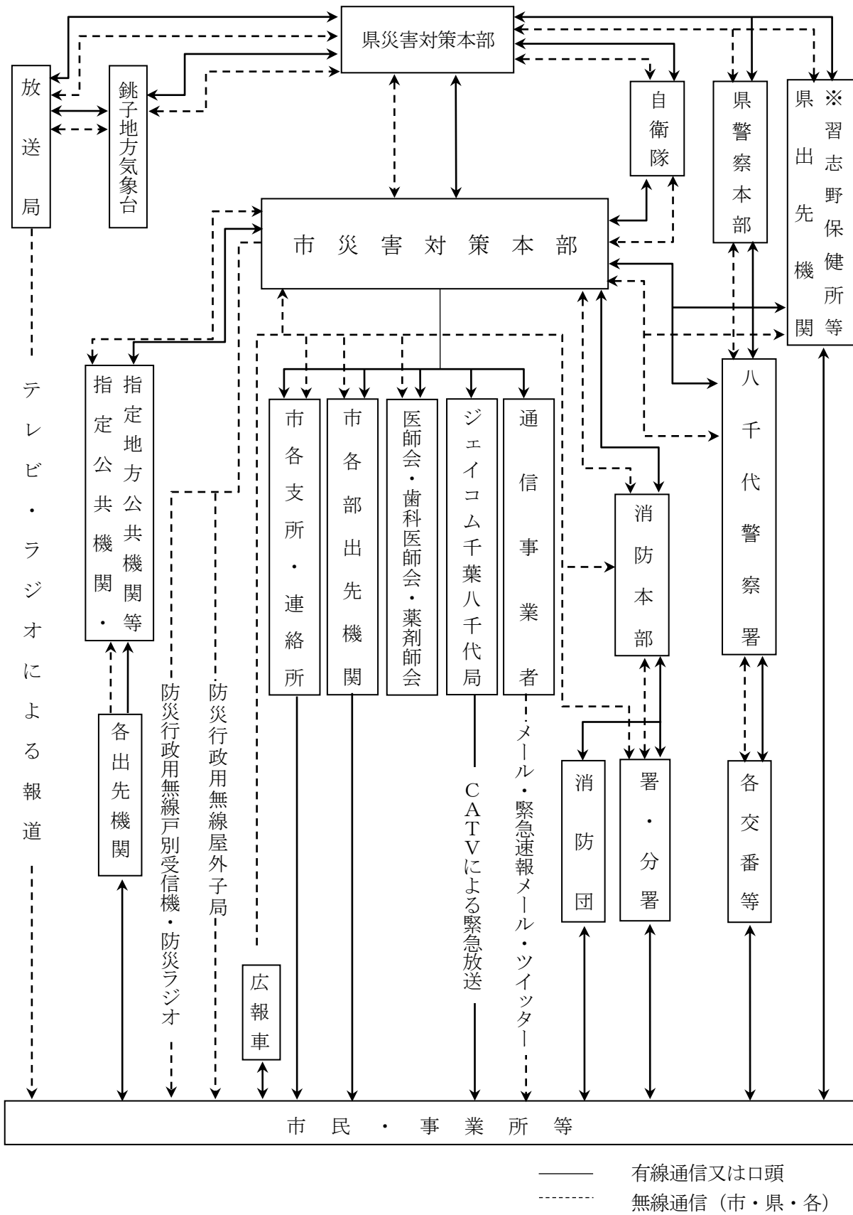
災害時の市本部を中心とする通信連絡系統図
